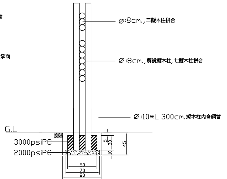
解說牌側立面圖
