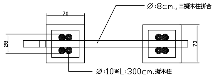
解說牌平面圖
