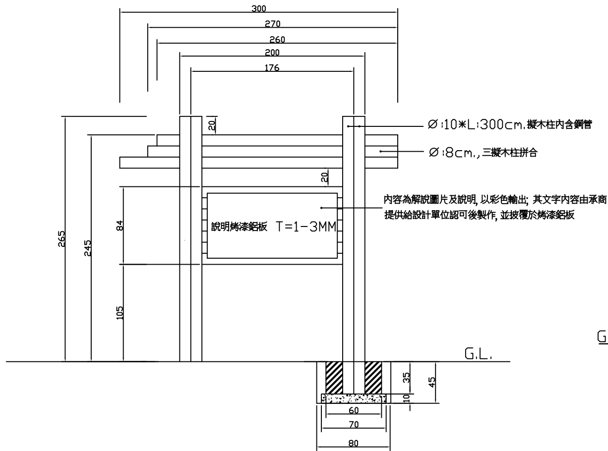
解說牌詳圖 (計4座)
