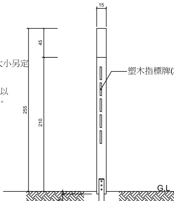
統一招牌側立面圖 Scale: 1/30 ref: 全區
