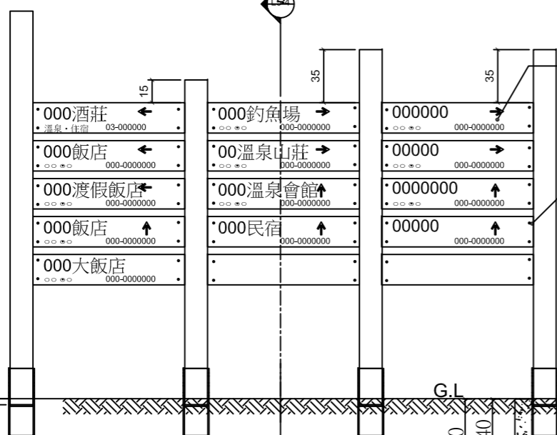
統一招牌立面圖 Scale: 1/30 ref: 全區
